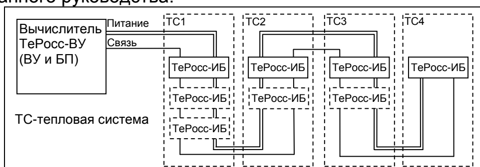
Рисунок 3.1. Структурная схема прибора ТеРосс
